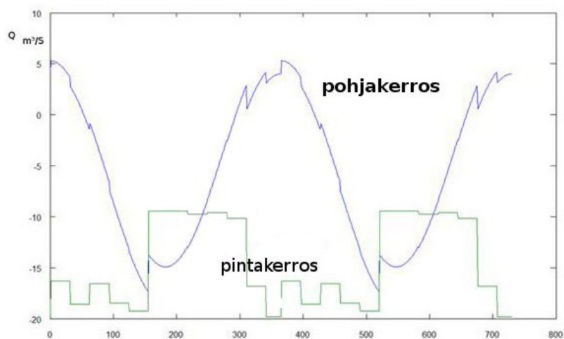
Kuva 3.53. Mallin laskema veden virtaama Tammisaaren salmien läpi ylä- ja alavedessä.
