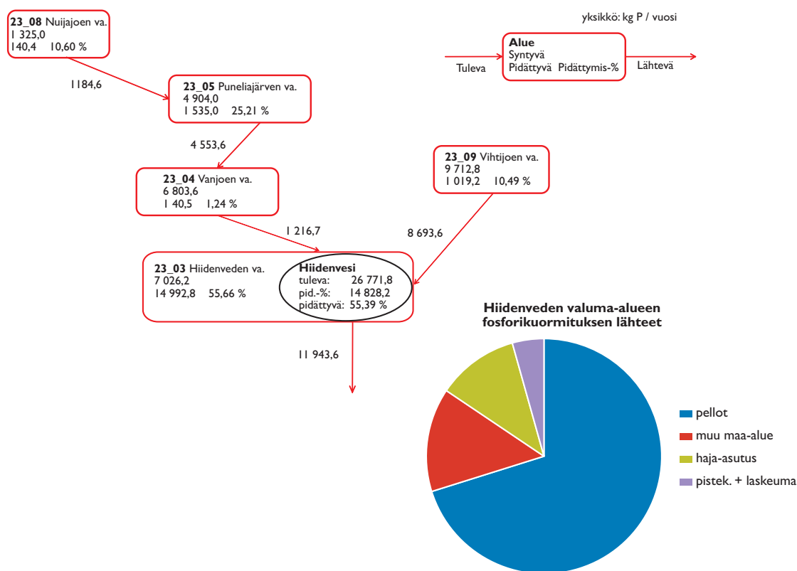
Kuva 3.7. Hiidenveden koko valuma-alueen fosforitasekaavio.
