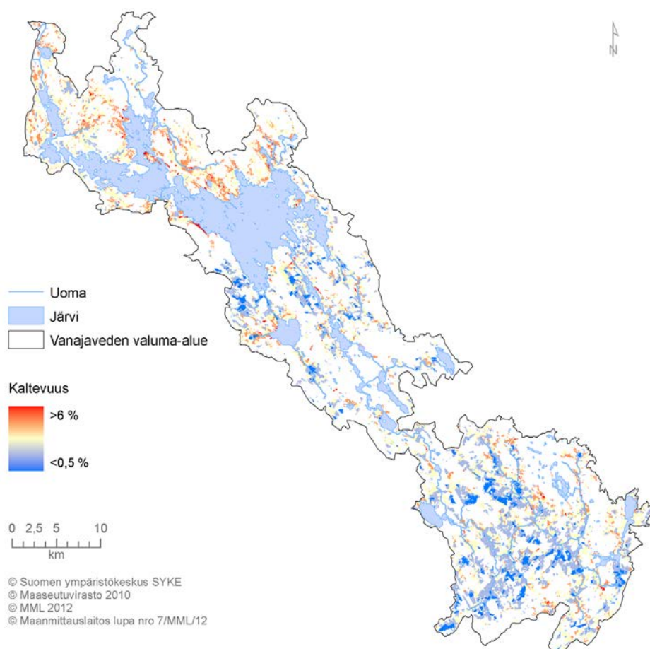
Kuva 3.60. Vanajaveden pilottialueen peltojen kaltevuus.
