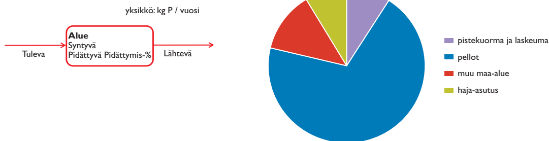
Kuva 3.64. Vanajanselän koko valuma-alueen fosforitasekaavio.
