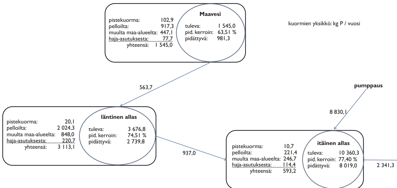
Kuva 3.30. Läntisen Pien-Saimaan valuma-alueen fosforitasekaavio – perustilanne.
