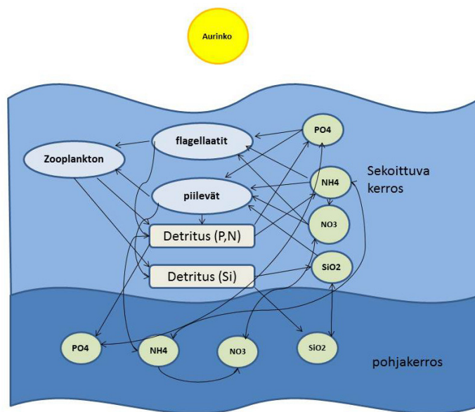
Kuva 3.54. Ekosysteemi- ja ravinnekiertomallin kaavio.
