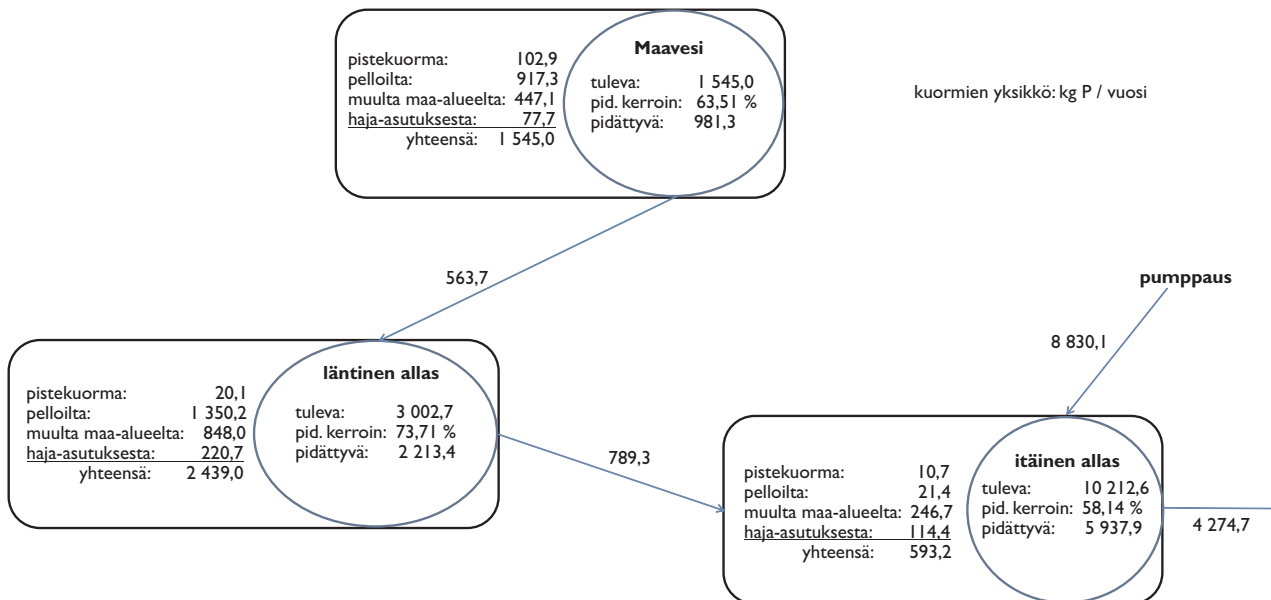
Kuva 3.31. Läntisen Pien-Saimaan valuma-alueen fosforitasekaavio – skenaario.
