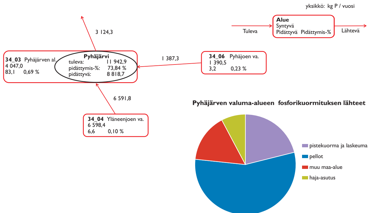
Kuva 3.45. Pyhäjärven koko valuma-alueen fosforitasekaavio.
