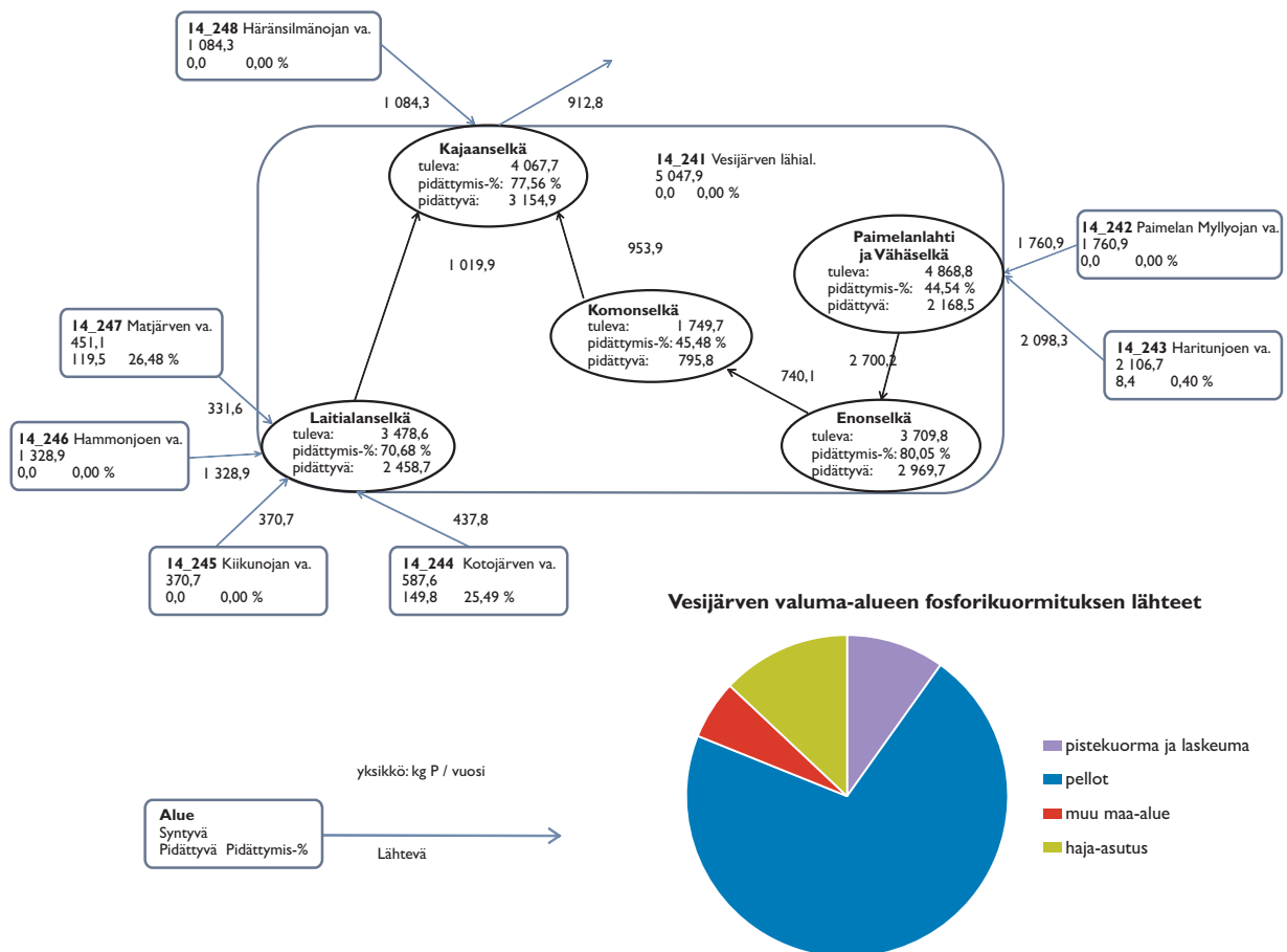
Kuva 3.94. Vesijärven valuma-alueen fosforitasekaavio, nykytilanne.
