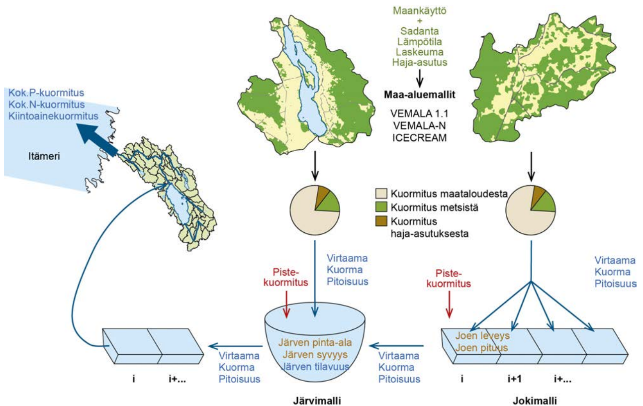
Kuva 2.2. WSFS-DEMOLA mallin perusrakenne.
